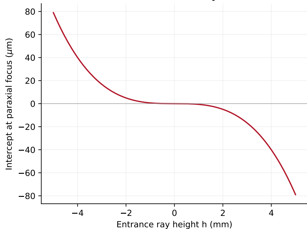
Exact refracted-ray fan
